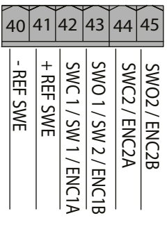
Intrări codificator/limitator
