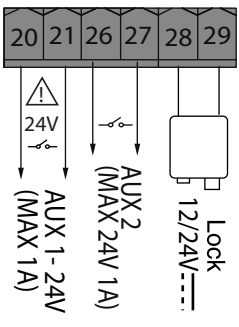
AUX
