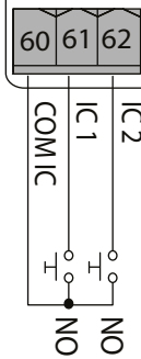
Comenzi
