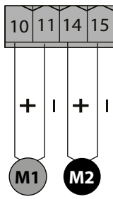
Motor
